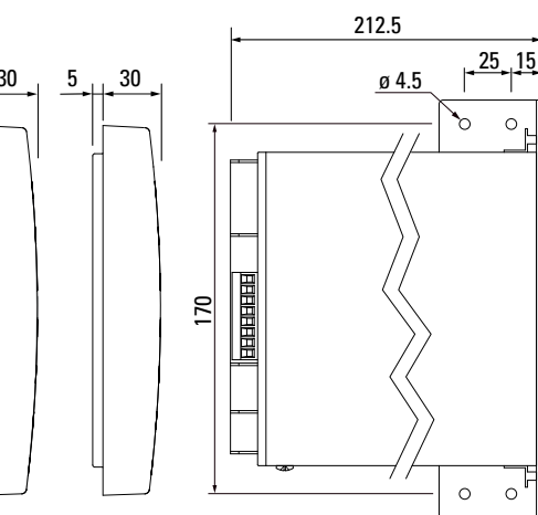
PANNELLO OPERATORE SEPARATO MONTAGGIO SPORGENTE (Pannello operatore separato)
