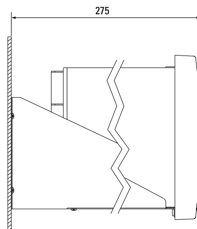
MONTAGGIO SPORGENTE
